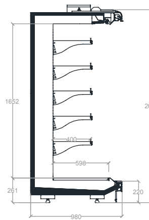
DRACO D22
