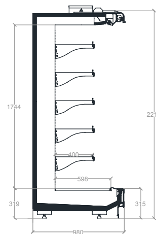
DORADO D32
