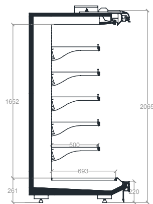
DRACO M22
