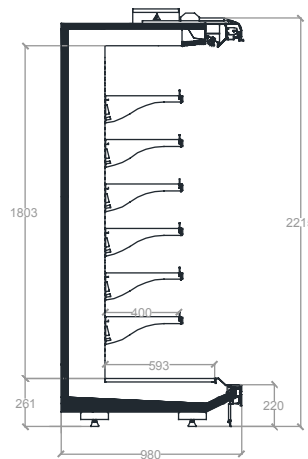
DORADO D22
